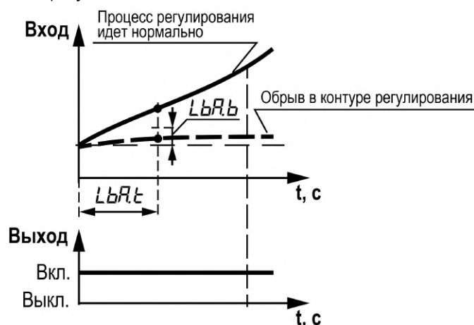
Рисунок 7.4 – Диагностика неисправности контура регулирования
