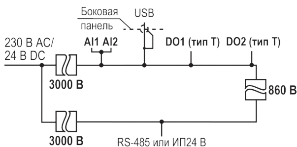
Рисунок 5.2 – Схема гальванической развязки (выход типа «Т»)
