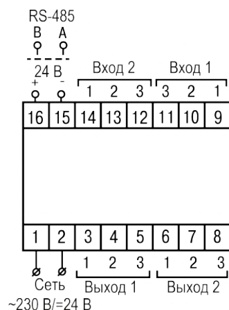
Рисунок 5.6 – Общая схема подключения 2TPM1–Д
