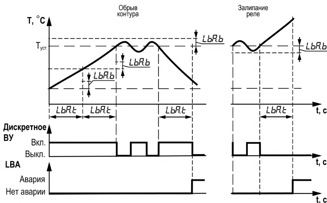
Рисунок 7.5 – Принцип работы диагностики обрыва контура регулирования
