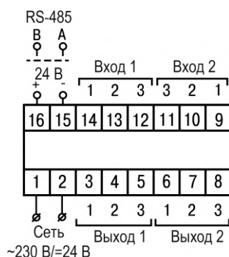
Рисунок 5.5 – Общая схема подключения 2TPM1–Щ5
