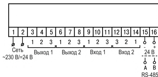
Рисунок 5.4 – Общая схема подключения 2TPM1–Щ1/Щ2
